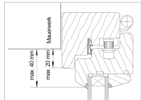
Sichtbare Rahmenbreite
