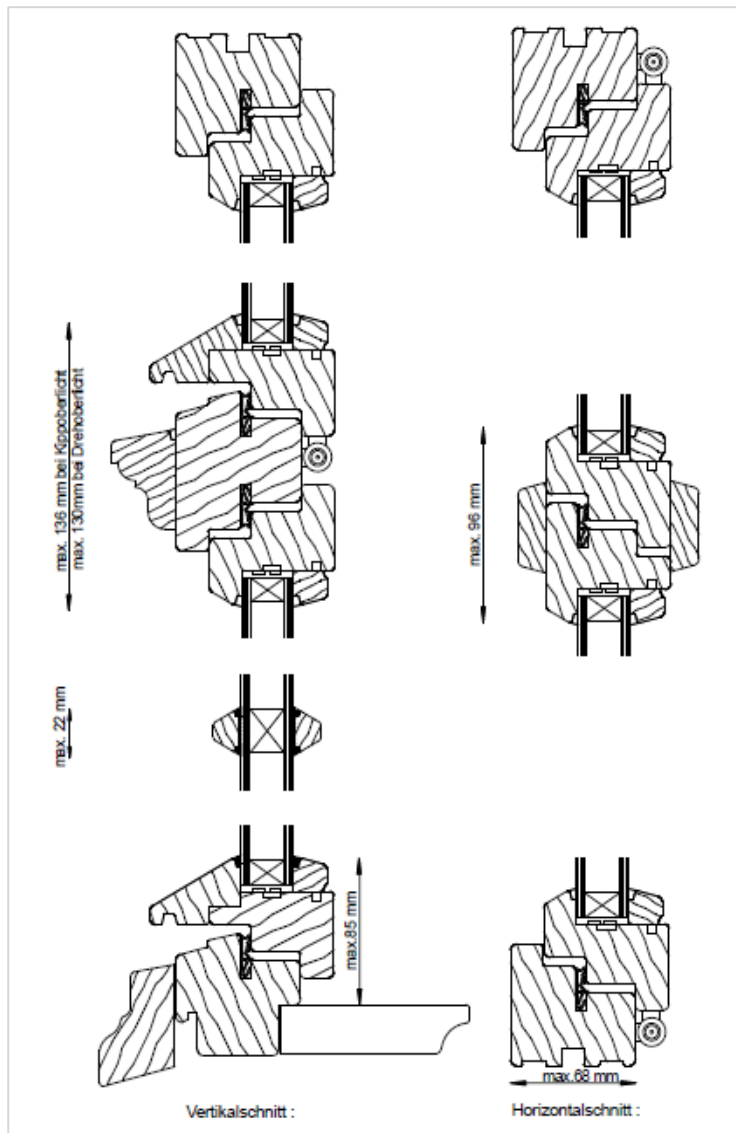
Sichtbare Rahmenbreite
