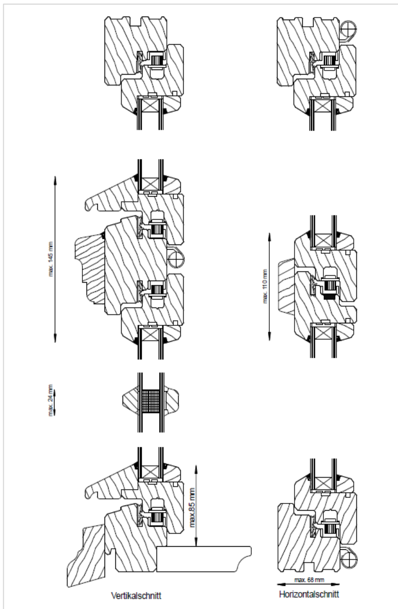
Sichtbare Rahmenbreite
